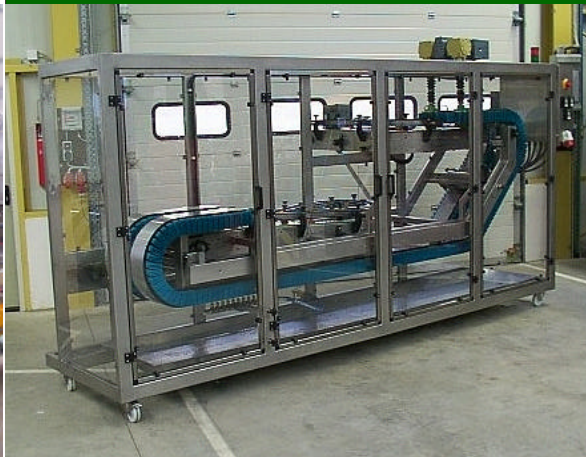
Rinser / Ausbläser / Flaschenwender
